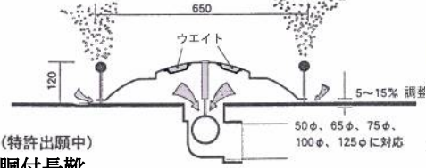
ユニット円水盤「UFO」65型
